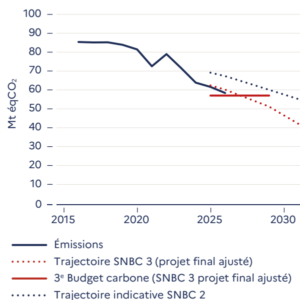
Figure 4.3.1.b – Émissions du secteur de l'industrie depuis 2015, budget carbone et trajectoire indicative du projet de SNBC 3 et trajectoire indicative de la SNBC 2
