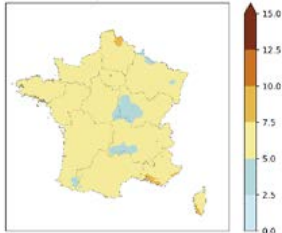
Moyenne annuelle des concentrations de PM_{2,5} ( \mu g/m^3 ) Scénario Citepa/BaseGES/QA+ 2050
