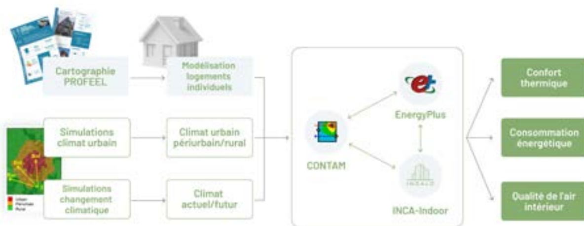
La chaîne de modélisation développée dans AMBRES
