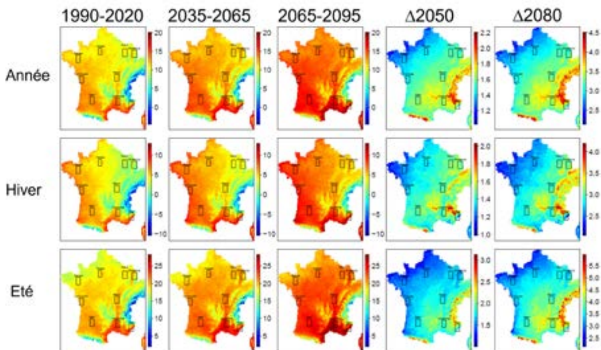
Cartes d'évolution de la température moyenne de l'air à 2 m (°C).
